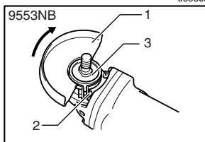
1. Protector de disco 2. Tornillo 3. Caja de cojinetes
